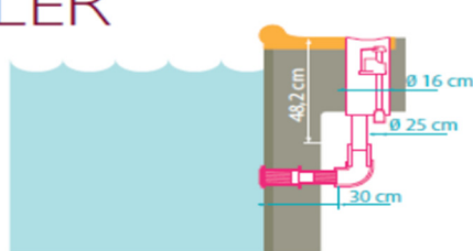
Régulateur de niveau
