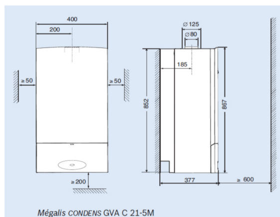
Mégalis CONDENS GVA C 21-5M
