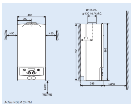
Acléis NGLM 24-7M
